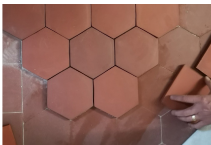
Carreaux carrés et hexagonaux; pièces spéciales: plinthes à gorge, plinthes à angle et coins arrondis
